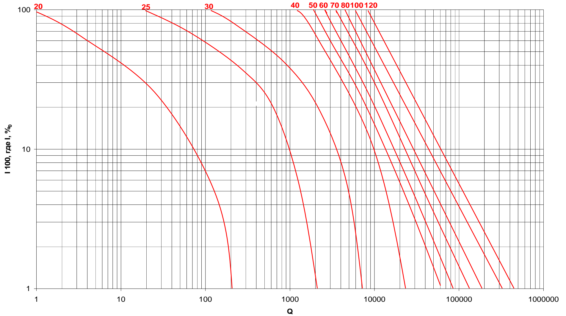
Рисунок 2 Определение соотношения \left(\frac{B}{h}\right)_{5\%}
